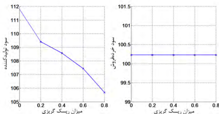
نمودار ۹. اثر میزان ریسک ( \lambda ) بر سود تولیدکننده و خرده‌فروش در مدل ۳
