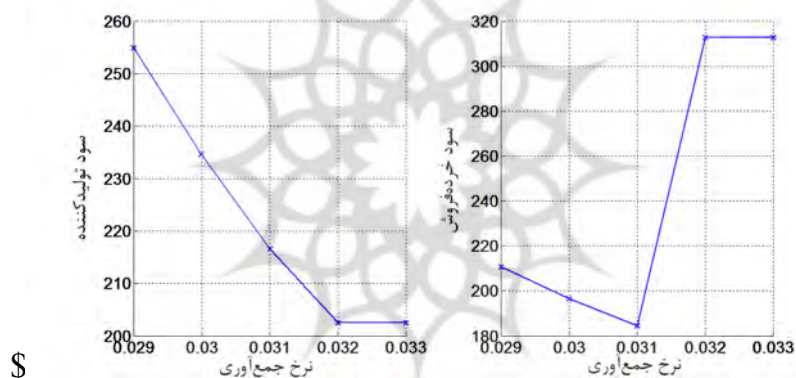
نمودار ۱. اثر نرخ جمع‌آوری ( \tau ) بر سود تولیدکننده و خریده‌فروش در مدل ۱
