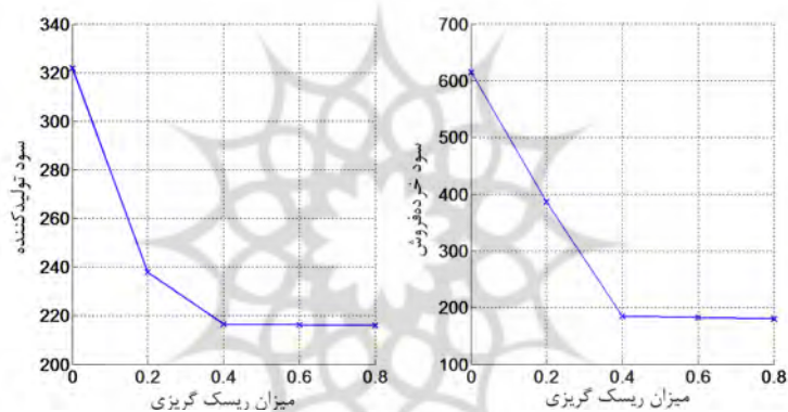
نمودار ۷. اثر میزان ریسک ( \lambda ) بر سود تولیدکننده و خرده‌فروش در مدل ۱
