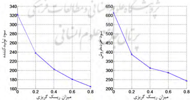
نمودار ۸. اثر میزان ریسک ( \lambda ) بر سود تولیدکننده و خرده‌فروش در مدل ۲
