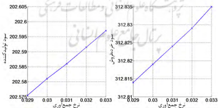
نمودار ۲. اثر نرخ جمع‌آوری ( \tau ) بر سود تولیدکننده و خریده‌فروش در مدل ۲
