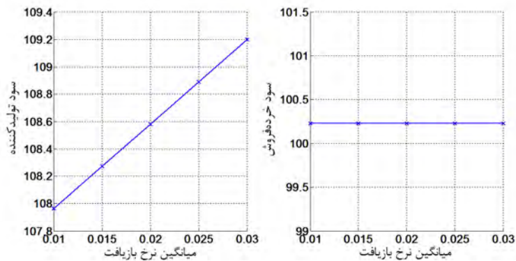
نمودار ۶. اثر میانگین نرخ بازیافت ( \bar{r} ) بر سود تولیدکننده و خرده‌فروش در مدل ۳
