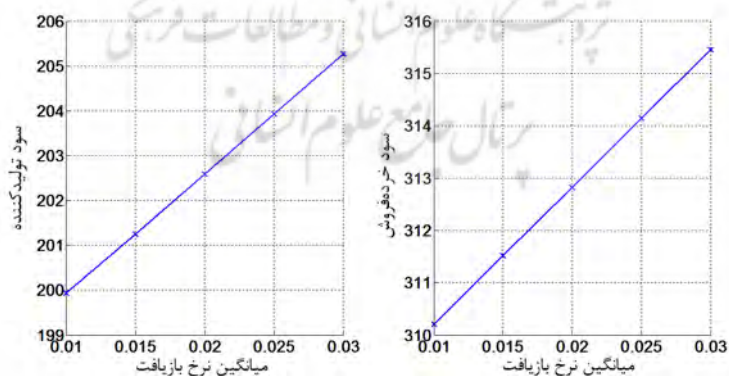
نمودار ۵. اثر میانگین نرخ بازیافت ( \bar{r} ) بر سود تولیدکننده و خردهفروش در مدل ۲
