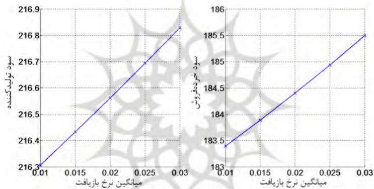
نمودار ۴. اثر میانگین نرخ بازیافت ( \bar{r} ) بر سود تولیدکننده و خردهفروش در مدل ۱
