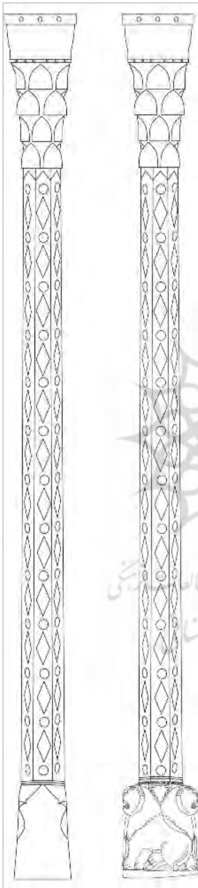
تصویر ۱۷. ستون‌های آیینه‌خانه همراه با تزئینات (نگارندگان، ۱۳۹۲)
