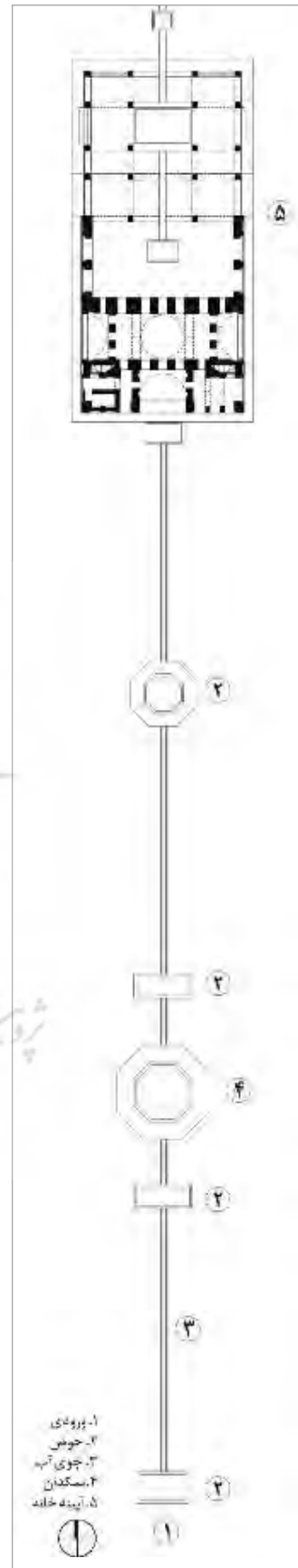
تصویر ۱۶. پلان آیینه‌خانه و موقعیت حوض‌ها در سایت (نگارندگان، ۱۳۹۲)
