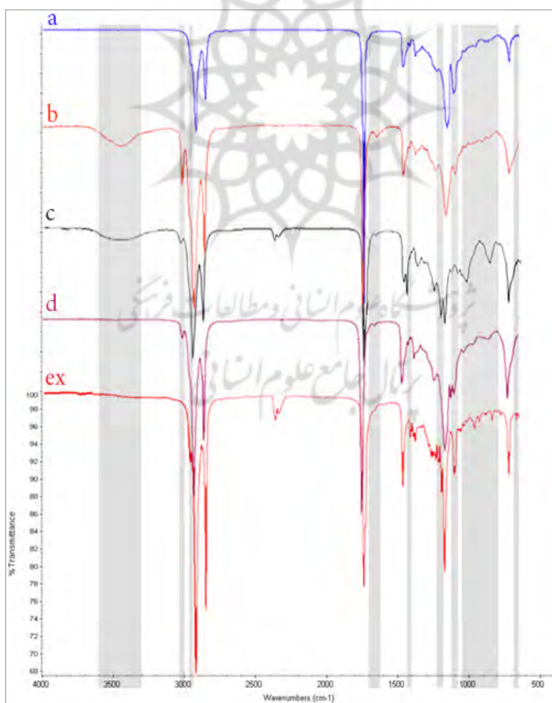
تصویر ۴. مقایسه طیف‌های ATR-FTIR انواع روغن گیاهی استفاده شده در روغن‌دهی چرم و روغن استخراجی. a: روغن نارگیل، b: روغن بزرک، c: روغن کرچک، d: روغن زیتون و ex: چرمی استخراجی از نمونه چرم (نگارندگان)
