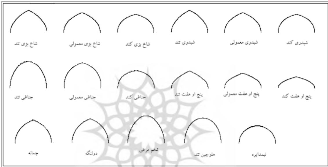
تصویر ۳. گونه‌هایی از چفدهای به‌کاررفته در معماری ایرانی، (تهیه و ترسیم از نگارندگان)
