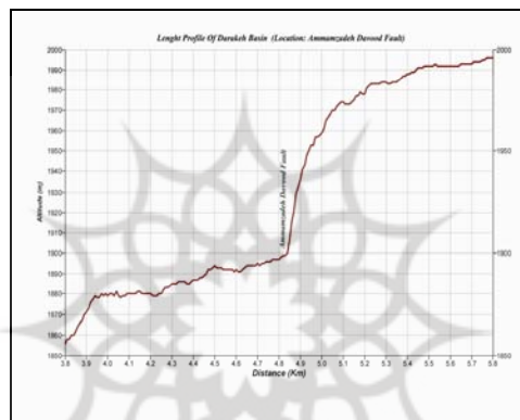
شکل ۷ نیمرخ طولی رودخانه درکه در محل گسل امامزاده داود مأخذ: نقشه توپوگرافی ۱/۵۰۰۰۰ تجریش، محاسبات نگارنده
