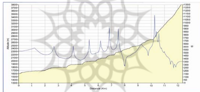
شکل ۱۸ تغییرات SL در امتداد نیمرخ طولی رودخانه اصلی در که مأخذ: نگارنده
