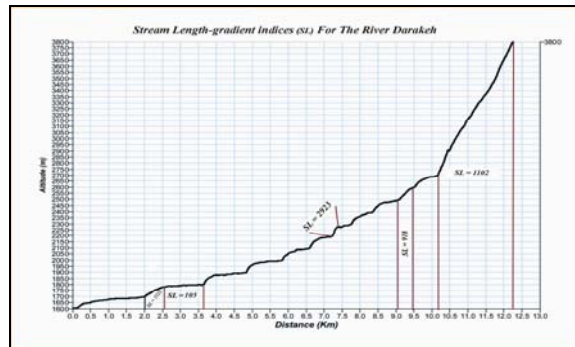
شکل ۶ برآورد شاخص SL در مناطق مشخص شده در امتداد نیمرخ طولی رودخانه درکه مأخذ: نمودار فوق بر اساس داده‌های حاصل از نقشه توپوگرافی ۱/۵۰۰۰۰ تجریش و محاسبات نگارنده و به کمک نرم افزار اکسل رسم شده است.
