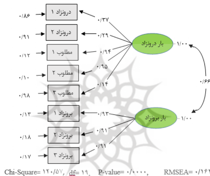
شکل ۳- مدل تحلیل عاملی تأییدی بار شناختی با ترکیب بعد درونزاد و مطلوب در حالت ضرایب استاندارد
