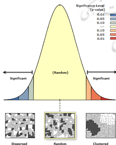
شکل ۴. الگوی فضایی روستاهای نمونه از نظر ظرفیت سازگاری در مقابل خشکیدن دریاچه ارومیه بر اساس تابع مورن (I)، منبع: نگارندگان، ۱۳۹۹
