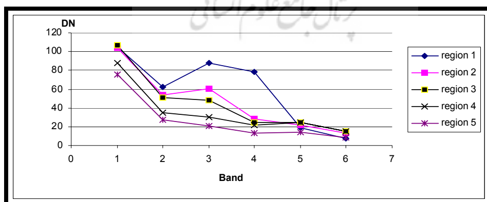
تصویر ۲- محدوده های انتخاب شده برای بررسی حساسیت باندهای TM به پارامترهای کیفی
