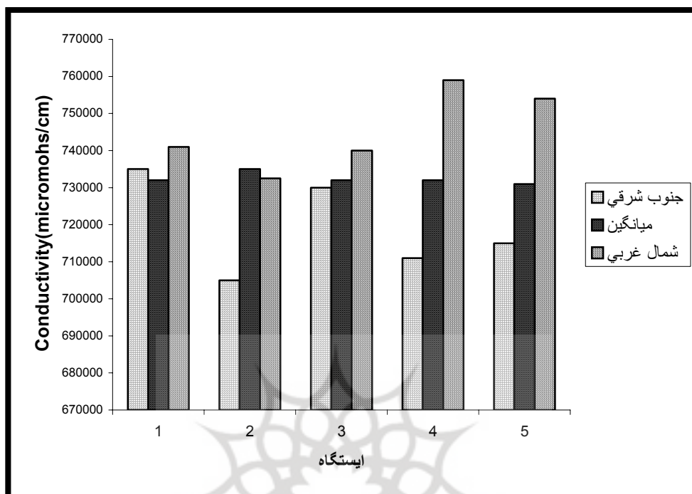
تصویر ۱- تغییرات میزان قابلیت هدایت الکتریکی آب دریاچه ارومیه در ایستگاه های پنجگانه جنوبشرقی و شمالغربی بزرگراه شهید کلانتری در مقایسه با میانگین کل ایستگاه ها در تاریخ ۱۳۸۰/۱۰/۲۵ (احمدی، محمد رضا ۱۳۸۱)
