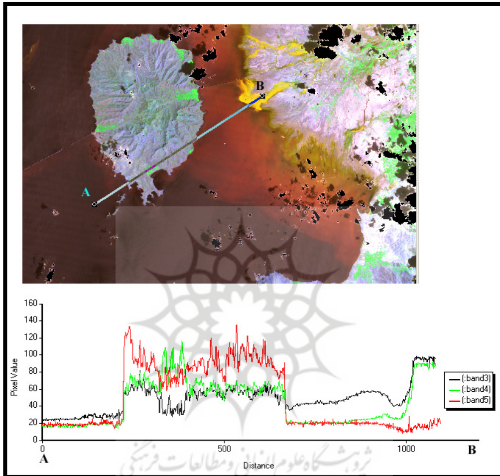
تصویر ۶- پروفیل طیفی تهیه شده در امتداد خط AB که بیانگر رفتار متفاوت باز معلق وارد شده از تلخه رود با سایر بخش های دریاچه به ویژه در باند (۵) می باشد.
