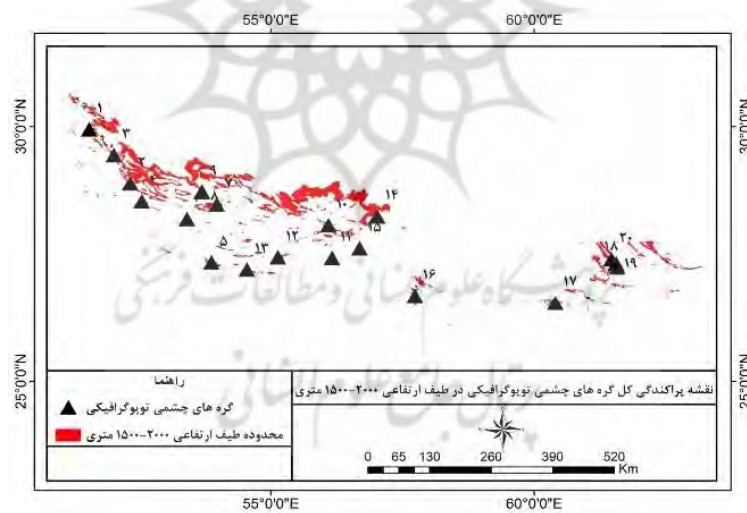
شکل - ۱۰: پراکندگی گره‌های چشمی توپوگرافیک در طیف ارتفاعی ۱۵۰۰-۲۰۰۰ متر
