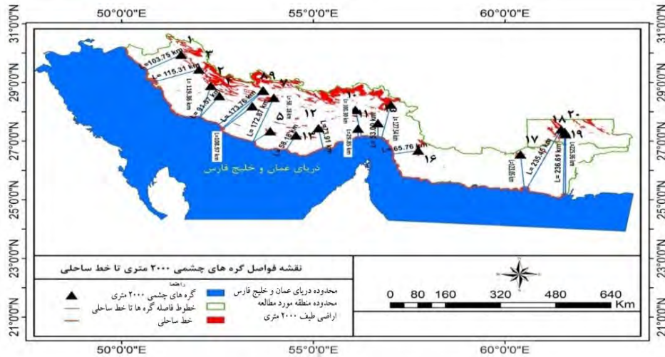
شکل - ۱۱: نقشه گره‌های چشمی با توجه به فاصله آنها با خط ساحلی
