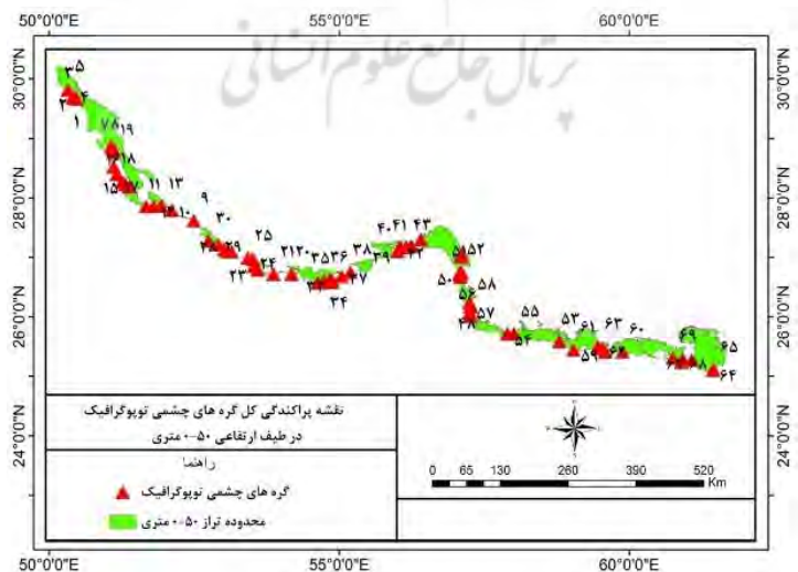
شکل - ۴: پراکندگی گره‌های چشمی توپوگرافیک در طیف ارتفاعی ۵۰-۰ متر
