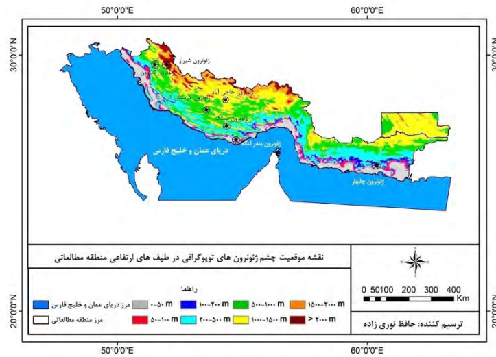
شکل - ۳: نقشه پهنه‌بندی طیف‌های ارتفاعی منطقه مطالعاتی
