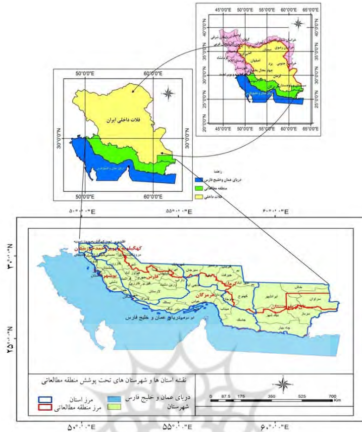
شکل - ۱: نقشه موقعیت منطقه پژوهش
