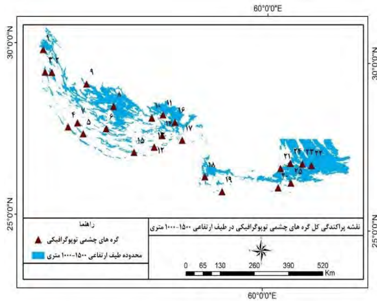
شکل - ۹: پراکندگی گره‌های چشمی توپوگرافیک در طیف ارتفاعی ۱۰۰۰-۱۵۰۰ متر
