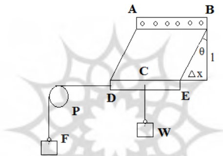
شکل ۲. شماتیک روش تیلور [۳۱]
