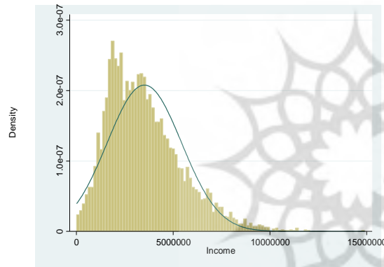
نمودار ۴- تابع چگالی احتمال درآمد فرد
