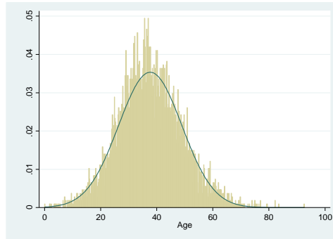
نمودار ۱- تابع چگالی احتمال سن افراد
