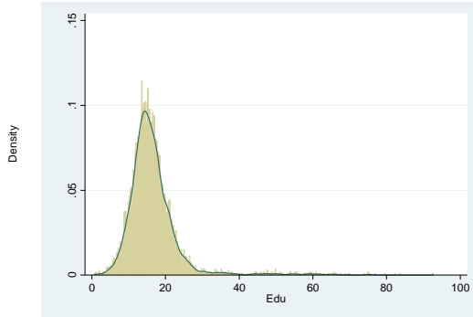
نمودار ۲- تابع چگالی احتمال تحصیلات افراد
