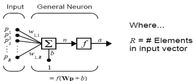
شکل ۲- مدل نرون در یک شبکه عصبی مصنوعی
