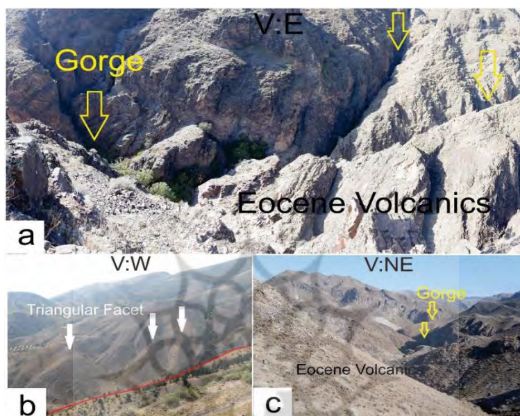
شکل ۱۴: لندفرم‌های مرتبط با فعالیت زمین‌ساختی گسل منجیل. (a) تنگ‌دره (Gorge) و حفر عمیق رودخانه در حوضه شماره ۵ (b) سطوح مثلثی ایجاد شده در اثر فعالیت گسل منجیل (c) تنگ‌دره (Gorge) در حوضه شماره ۷
