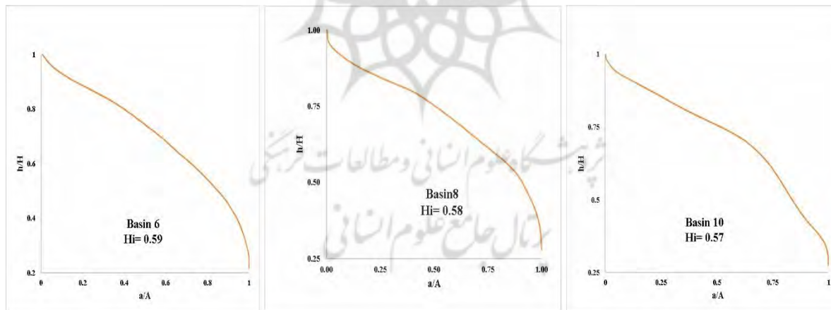
شکل ۷: منحنی بیشینه فرازسنجی در حوضه‌های شماره ۶، ۸ و ۱۰
