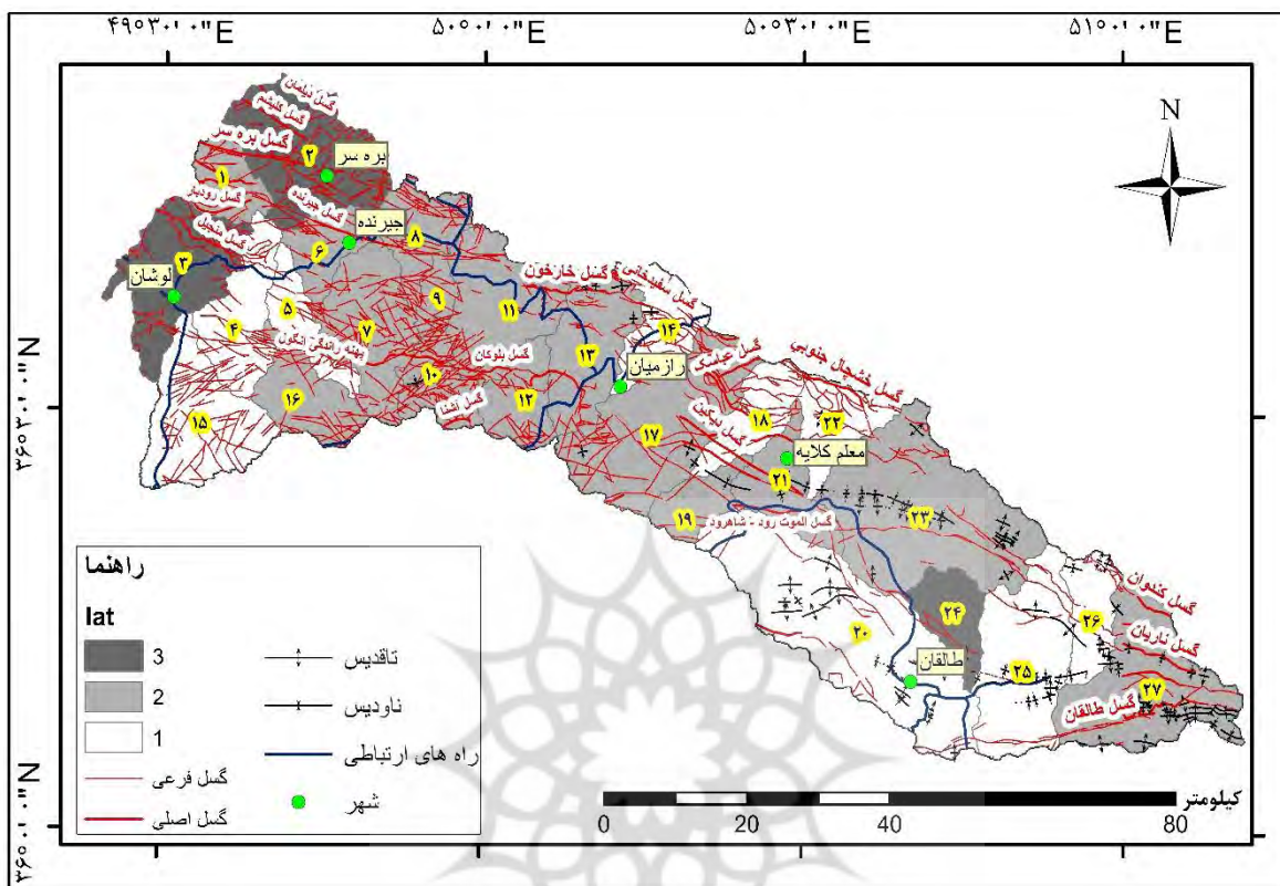
شکل ۱۲: نقشه توزیع سطح فعالیت زمین‌ساختی نسبی (Iat) در گستره مطالعاتی.
