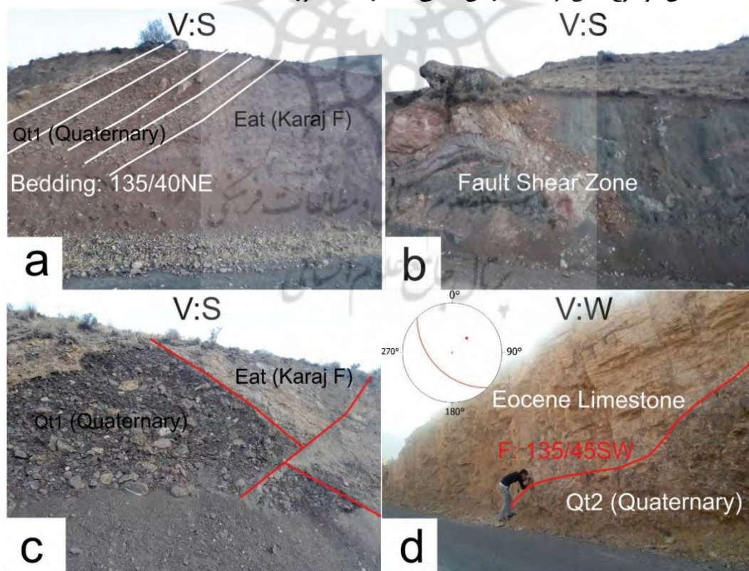
شکل ۱۳: دگرشکلی های ایجاد شده در واحدهای کواترنری. (a) کج شدگی واحدهای پادگانه ابرفتی تحت تاثیر فعالیت گسل انگول و نهشته شدن آن ها به صورت دگرشیب بر روی سازند کرج، (b) پهنه برشی گسل با حدود ۲۰ متر عرض در حوضه شماره ۱۱، (c) گسلش در پادگانه ابرفتی و راندگی سازند کرج بر روی آن در حوضه شماره ۷، (d) گسلش در واحدهای کواترنری تحت تاثیر گسل جیرنده.
