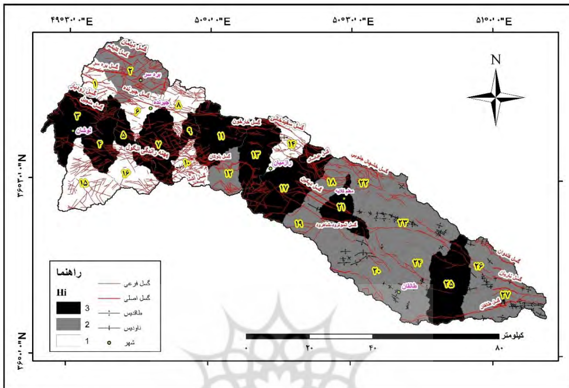
شکل ۶: نقشه رده‌بندی شاخص فرازسنجی در گستره مطالعاتی
