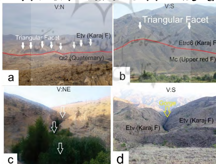
شکل ۱۵: لندفرم‌های مرتبط با فعالیت زمین‌ساختی اخیر در منطقه. (a) سطوح مثلثی مربوط به حوضه شماره ۱۲ تحت تاثیر فعالیت گسل منجیل و راندگی سازند کرج بر روی سازند قرمز بالایی بر اثر فعالیت گسل شاهرود (c) دره عمیق و تنگ در حوضه شماره ۸ که دارای رودشکن و نشان‌گر فعالیت گسل جیرنده است. (d) حفر قائم رودخانه در حوضه شماره ۱۲.
