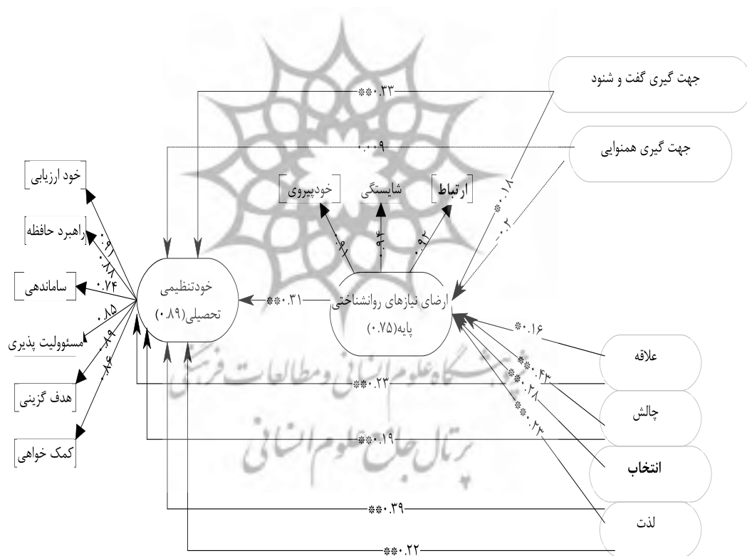
شکل ۲: مدل معادلات ساختاری در حالت ضرایب استاندارد
