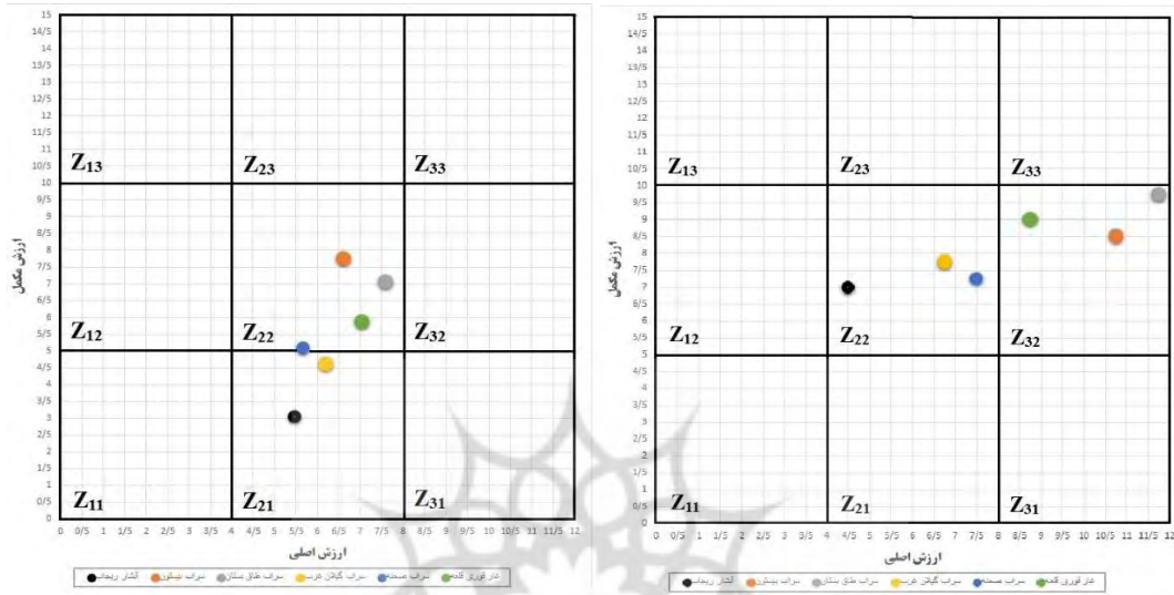
شکل ۲. موقعیت ژئومورفوسایت های ارزیابی شده با مدل های GAM (سمت راست) و مدل اصلاح شده GAM (سمت چپ)، منبع: نگارندگان، ۱۳۹۹
