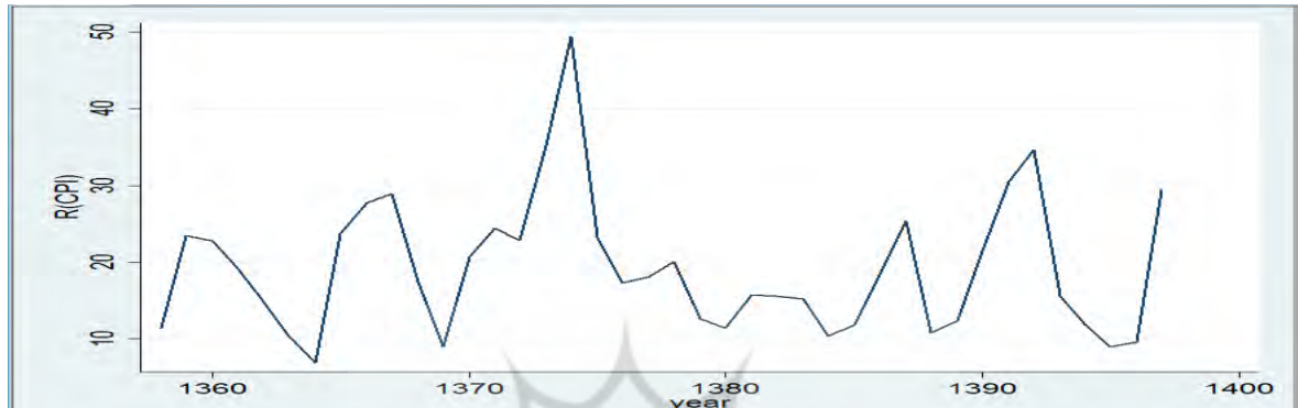
نمودار ۱- رشد سالانه شاخص قیمت مصرف‌کننده
