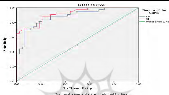
شکل ۱۰- منحنی نرخ پیش‌بینی نقشه‌های خطر زمین‌لغزش با استفاده از مدل‌های نسبت فراوانی و شاخص آماری
