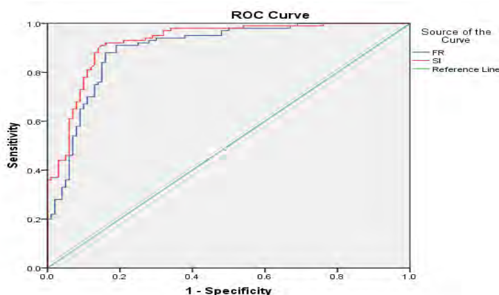
شکل ۹: منحنی نرخ موفقیت نقشه‌های خطر زمین‌لغزش با استفاده از مدل‌های نسبت فراوانی و شاخص آماری
