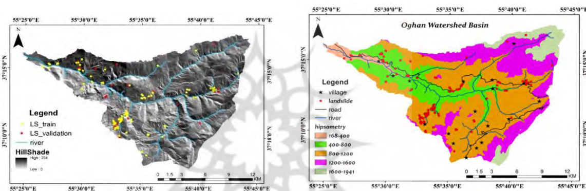
شکل ۳: موقعیت زمین لغزش‌های ثبت شده
