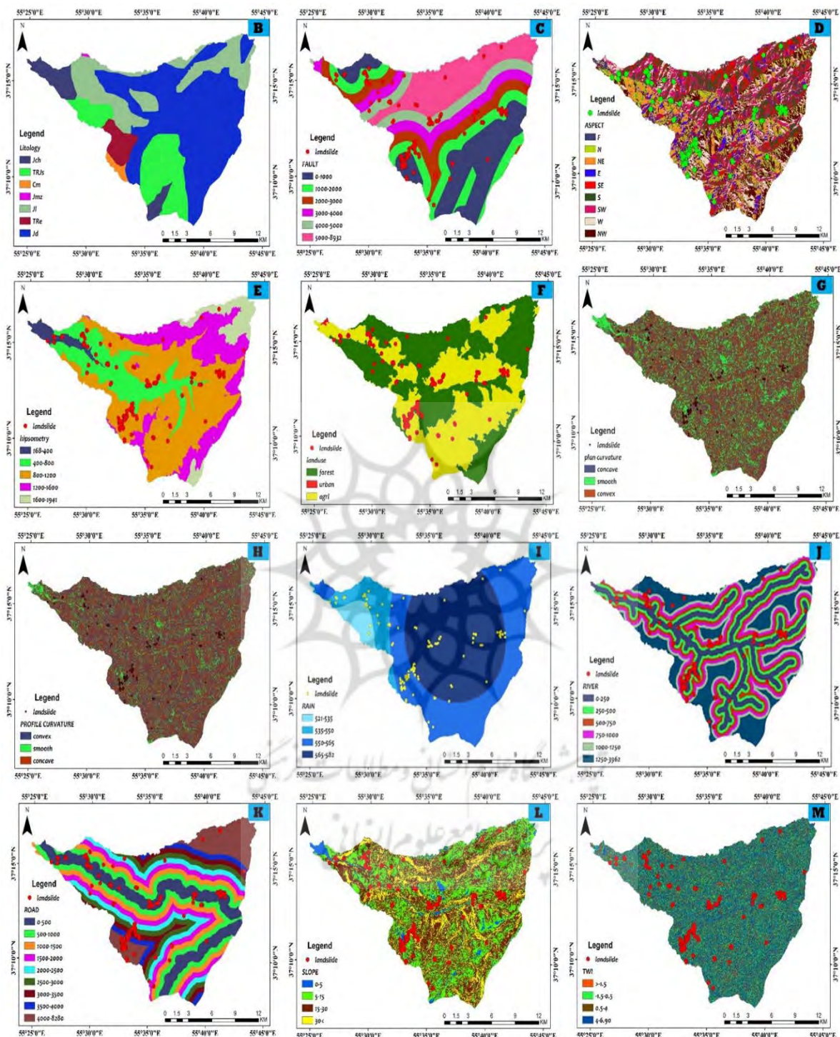
شکل ۵: نقشه‌های فاکتورهای مؤثر در بروز زمین‌لغزش به ترتیب: B (لیتولوژی)، C (فاصله از گسل)، D (جهت شیب)، E (ارتفاع)، F (کاربری اراضی)، G (انحنای طولی دامنه)، H (انحنای عرضی دامنه)، I (بارندگی)، J (فاصله از رودخانه)، K (فاصله از جاده)، L (شیب)، M (شاخص رطوبت توپوگرافی)
