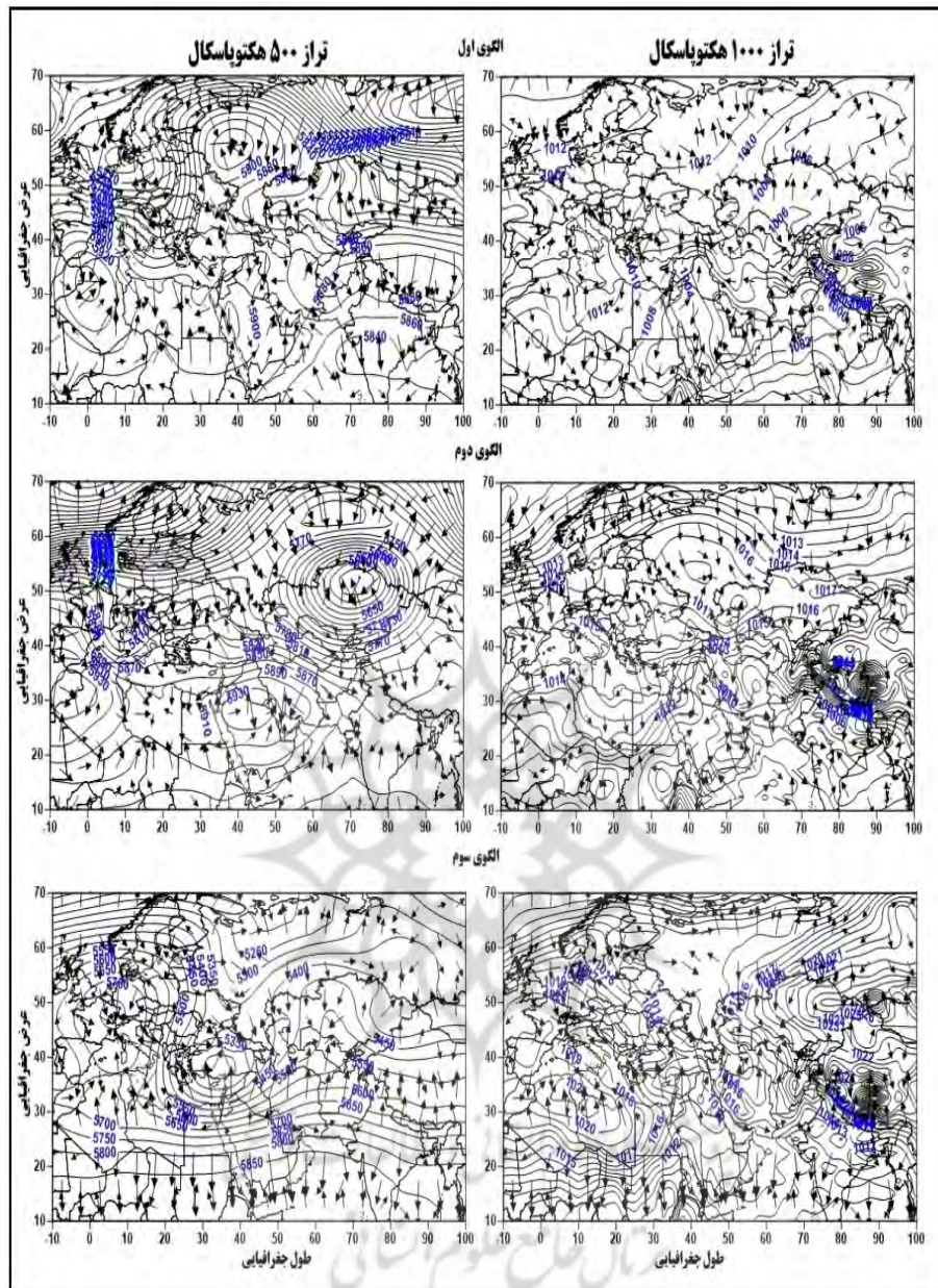
شکل (۴). الگوهای جوی فشار، ارتفاع و جهت باد برای روز نماینده در تراز ۵۰۰ و ۱۰۰۰ هکتوپاسکال
