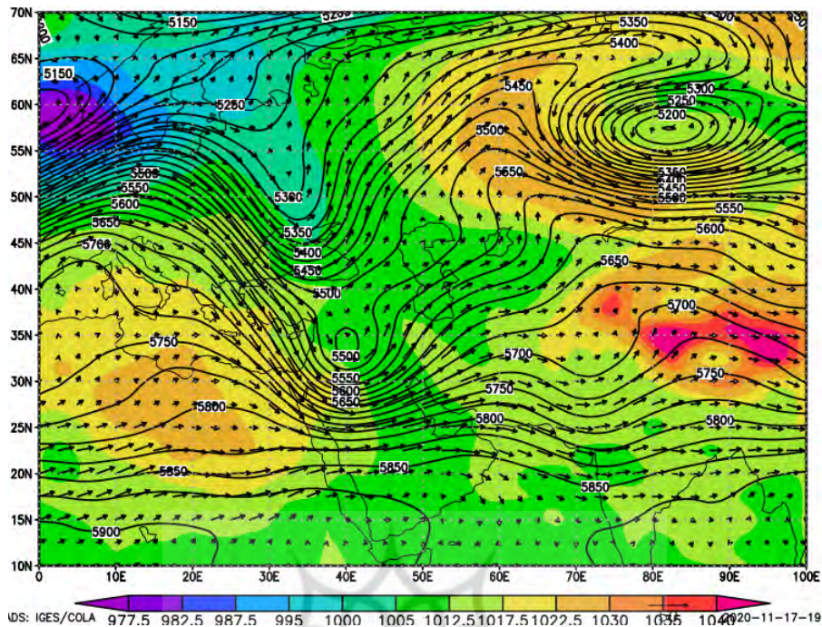
شکل ۳- نقشه ترکیبی فشار تراز دریا، ارتفاع ژئوپتانسیل (متر) تراز ۵۰۰ هکتوپاسکال و بردار باد تراز ۵۰۰ هکتوپاسکال ساعت صفر زولو روز ۲۶ اسفند ۱۳۹۷
