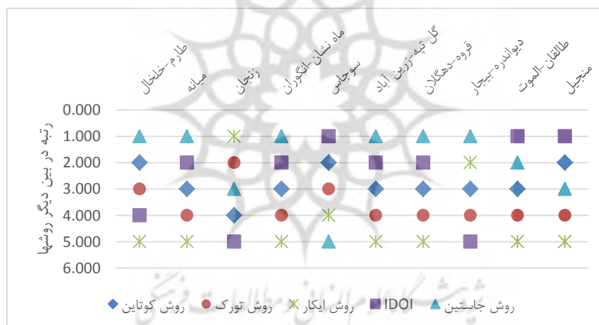
شکل ۲. رتبه روش‌های منتخب در مقایسه با یکدیگر از نظر ضریب همبستگی
