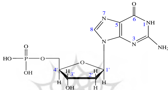
شکل ۸. نمای مولکولی گوانیلک اسید، H_7(5'-GMP)
