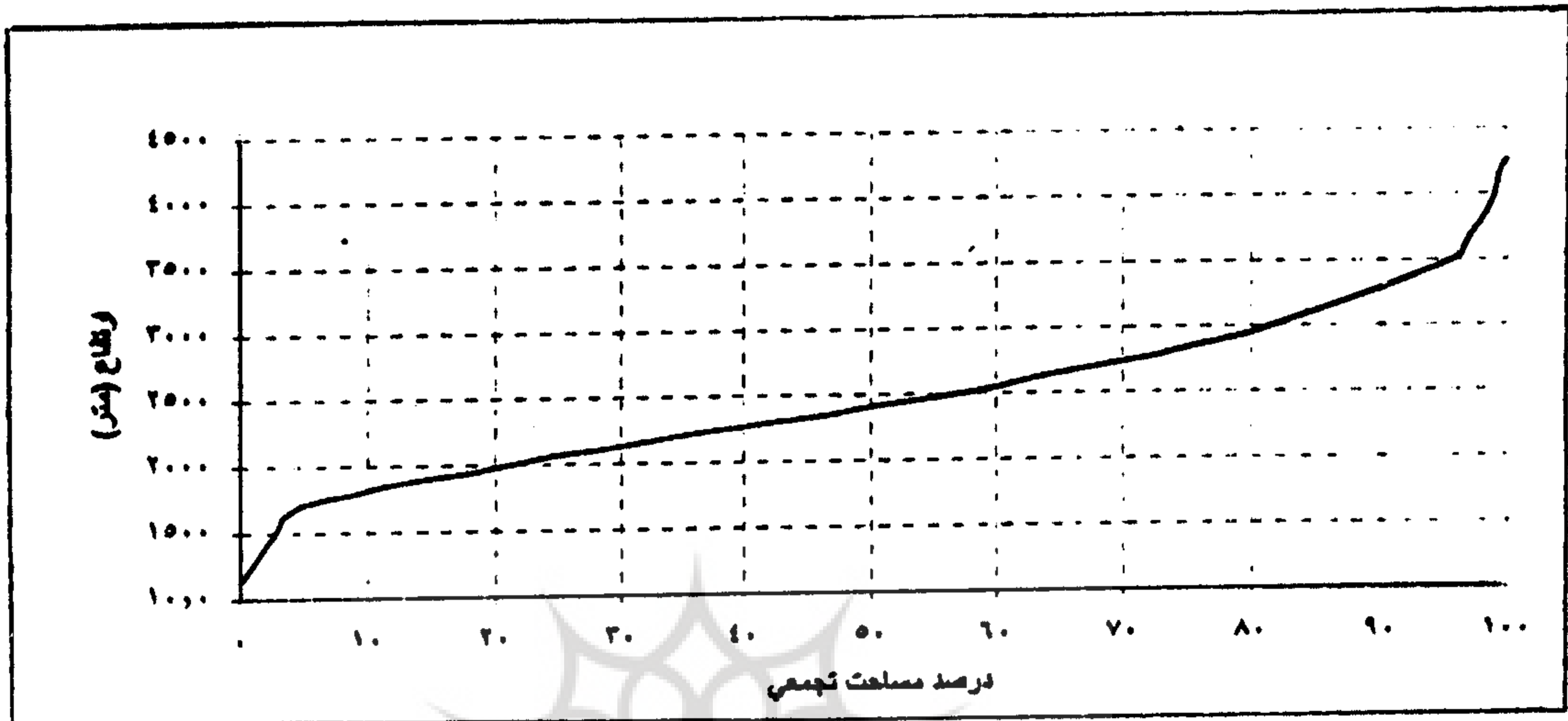
شکل ۱- منحنی تغییرات سطح با ارتفاع در حوضه آبریز طالقان (منحنی هیپسومتریک)
