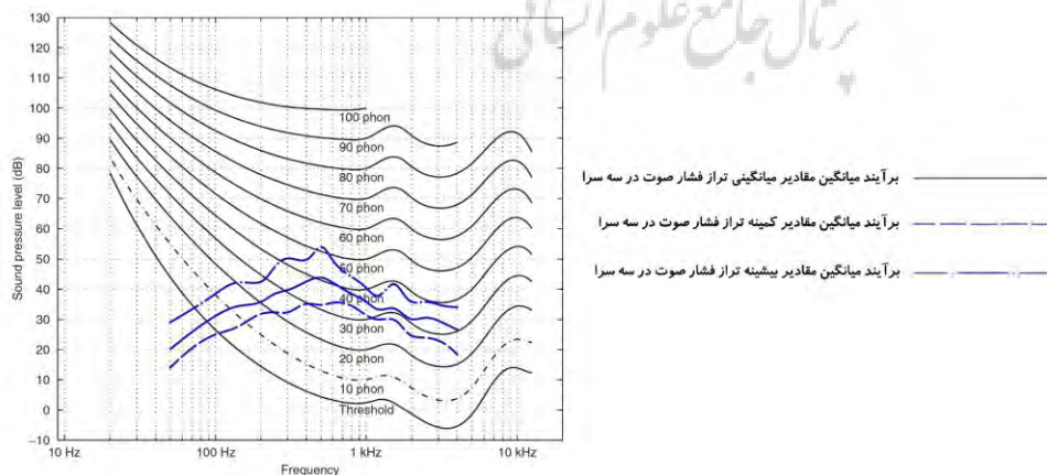
تصویر ۱۶: برآیند میانگین مقادیر کمینه، میانگین و بیشینه تراز فشار صوت در سه سراه نسبت به نمودار نرمال هم‌ترازی بلندی صدا
