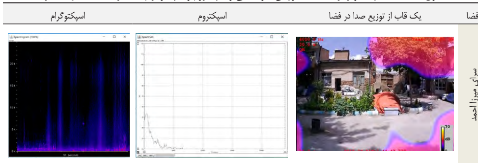
جدول ۶: یک قاب از تصاویر برداشت‌شده دوربین آکوستیکی و اسپکتروم و اسپکتوگرام نقاط برداشت‌شده در سه سرا
