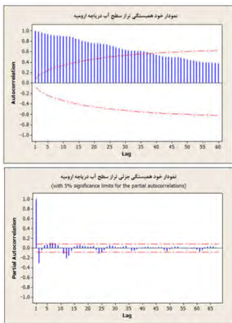
شکل (۵): نمودار ACF سری زمانی با نزول نمای
