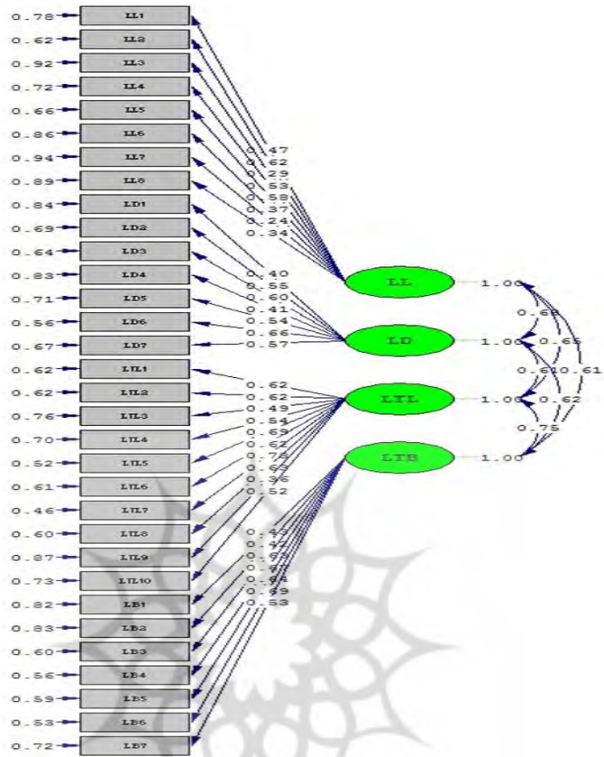
شکل (۱): تحلیل چهار عاملی برای مؤلفه‌های یادگیری پویا
