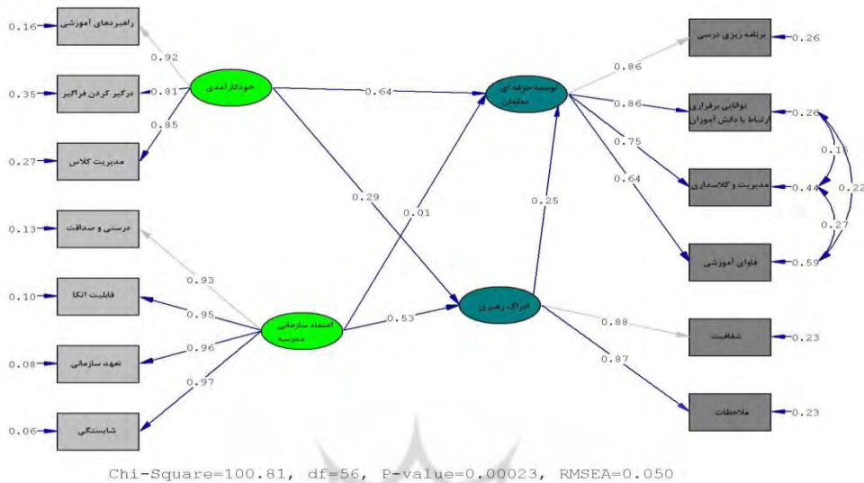
شکل ۲: نمودار مسیر مدل برازش شده همراه با پارامترهای برآورد شده (مقادیر استاندارد)
