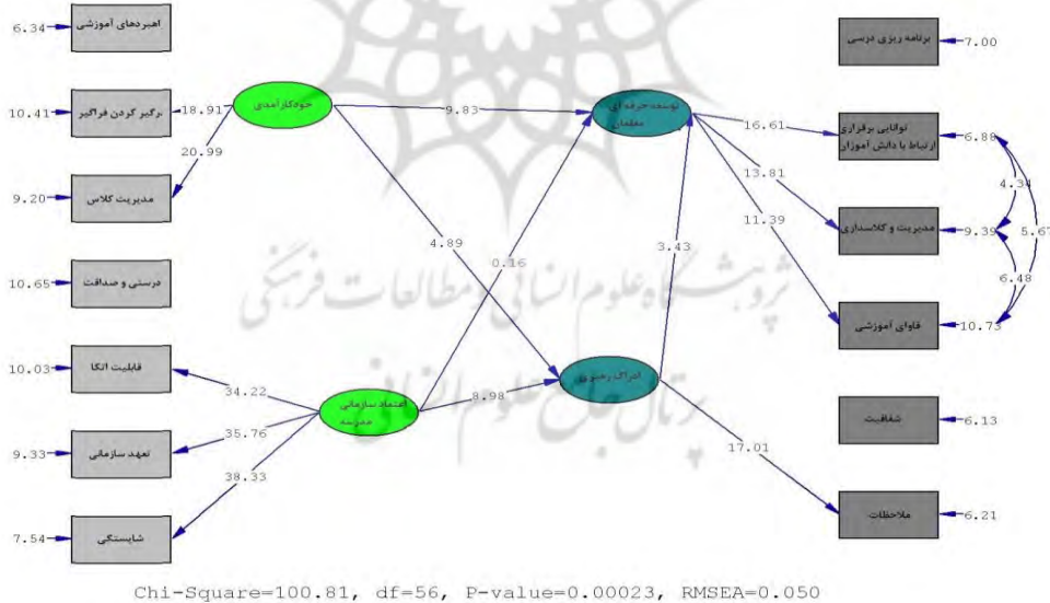
شکل ۳: نمودار مسیر مدل برازش شده همراه با پارامترهای برآورد شده (آماره t)
