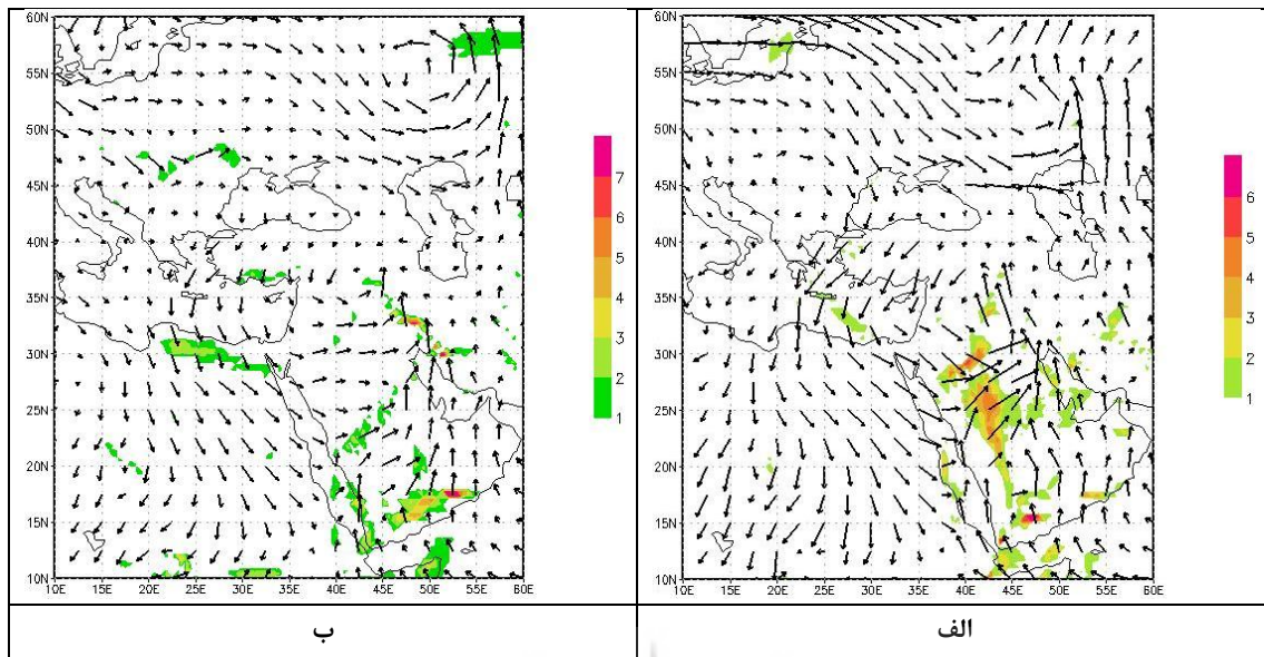
شکل ۱۱. نقشه وزش رطوبت بر حسب گرم بر کیلوگرم در ثانیه (در راهنمای نقشه به دلیل کوچک بودن مقادیر وزش اعداد در ۱۰ میلیون ضرب شده‌اند) (الف) ساعت ۱۸ روز ۲۴ مارس (ب) ساعت ۶ روز ۲۵ مارس در نتیجه‌ی الگوی جریان مشاهده شده، بیشینه‌ی رطوبت نسبی (بیش از ۹۰٪) و رطوبت ویژه در امتداد منطقه همگرایی دریای سرخ، غرب و جنوب ایران شکل گرفت (شکل ۱۲). به طوری که رطوبت ویژه در جنوب ایران در منطقه نسبتاً گسترده‌ای به بیش از ۰/۰۱ کیلوگرم در کیلوگرم رسید و در روز رخداده سیل (روز ۲۵ مارس) در بخش‌هایی از جنوب غرب ایران از مقدار ۰/۰۱ کیلوگرم در کیلوگرم فراتر رفت. در روزهای بعد به تدریج با تغییر وزش جریانات، منطقه‌ی بیشینه رطوبت به سمت شرق جابجا شد.
