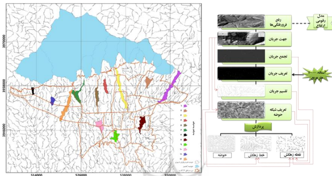
شکل ۴: نقشه پراکنش حوضه‌های هیدرولوژی شهری نمونه در شهر تهران
