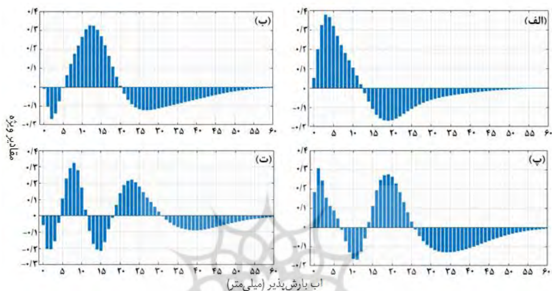
شکل ۲. نمودار مقادیر ویژه هر یک از مؤلفه‌ها. محور افقی مقدار آب بارش‌پذیر به میلی‌متر و محور عمودی مقادیر ویژه‌اند
