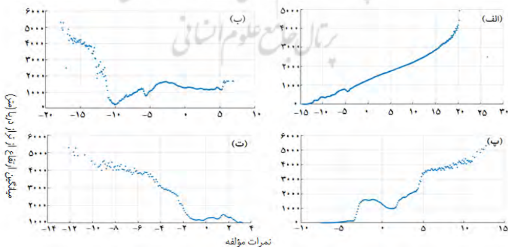
شکل ۴. رابطه ارتفاع از تراز دریا و مؤلفه‌های اصلی. الف) مؤلفه اول؛ ب) مؤلفه دوم؛ پ) مؤلفه سوم؛ ت) مؤلفه چهارم. محور افقی نمرات مؤلفه و محور عمودی میانگین ارتفاع از تراز دریا به متر
