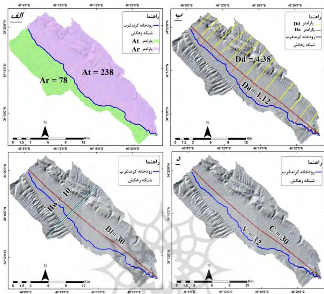
شکل ۴. محاسبه شاخص‌های مورفولوژیک و پارامترهای آن‌ها در حوضه کرند غرب؛ الف) شاخص عدم تقارن در حوضه کرند غرب (AF)؛ ب) شاخص تقارن توپوگرافی عرضی (T) در حوضه کرند غرب؛ ج) شاخص شکل حوضه (Bs) در حوضه کرند غرب؛ د) شاخص سینوزیته رودخانه (S) در حوضه کرند غرب
