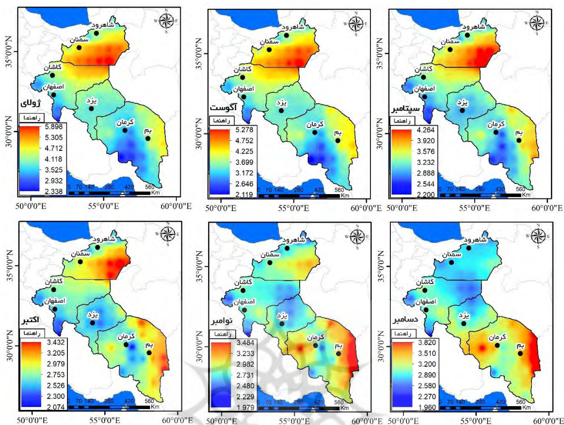
شکل ۴. پراکنش مکانی باد (m/s) در ایران مرکزی براساس پایگاه داده‌های نسخه ERA-Interim
