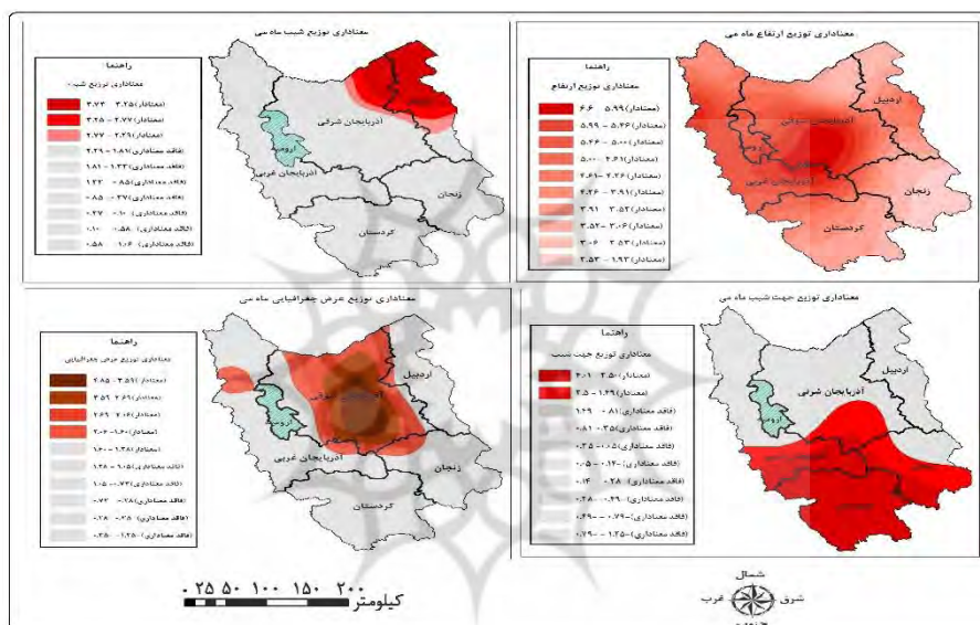
شکل ۵. توزیع آماره T برای هر متغیر مستقل (جهت شیب، ارتفاع، شیب، عرض جغرافیایی) در ماه می
