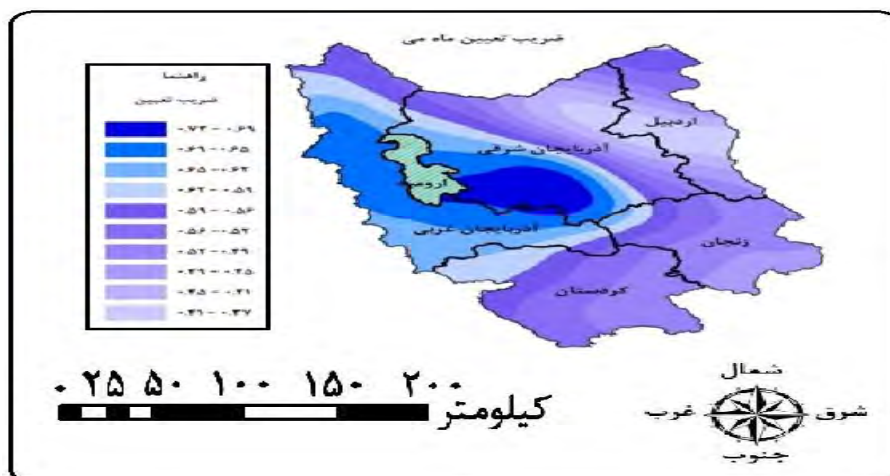
شکل (۶). ضریب تعیین مدل رگرسیون وزن دار جغرافیایی در ماه می
