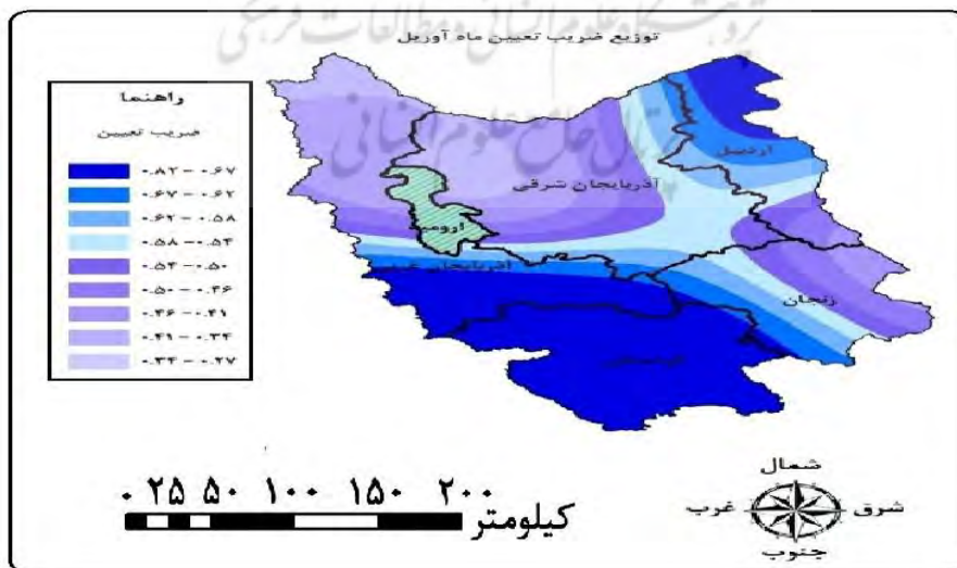
شکل (۴). ضریب تعیین مدل رگرسیون وزن دار جغرافیایی در ماه آوریل
