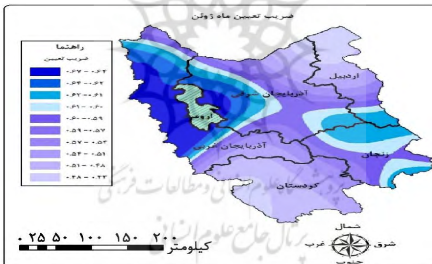
شکل (۸). ضریب تعیین مدل رگرسیون وزن دار جغرافیایی در ماه ژوئن
