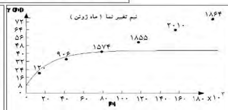
شکل (۲) نمودار نیم تغییرنمای برازش داده شده در سه ماه آوریل، می و ژوئن
