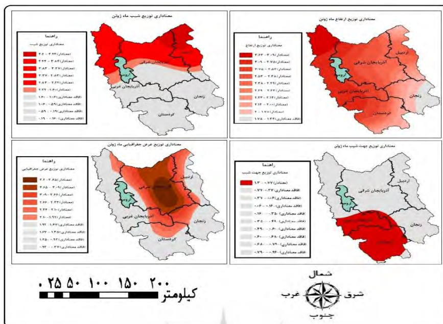
شکل (۷). توزیع آماره T برای هر متغیر مستقل در ماه ژوئن
