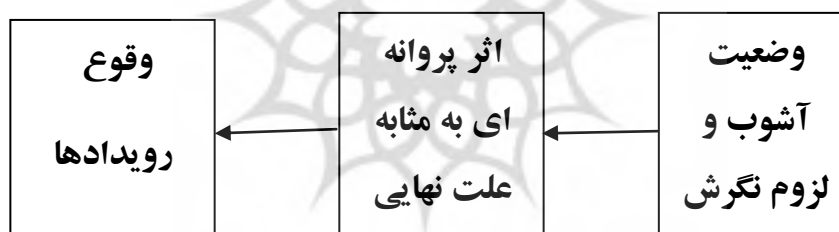
شکل ۲- مدل نظری
