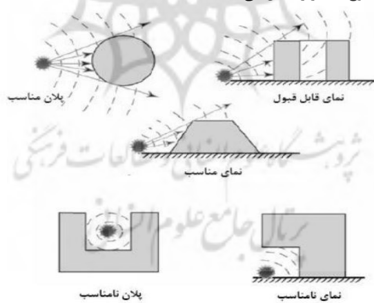
شکل ۱۹_ تأثیر شکل ساختمان در پلان و نما در برابر موج انفجار، ماخذ: (مبحث ۲۱ مقررات ملی ساختمان).
