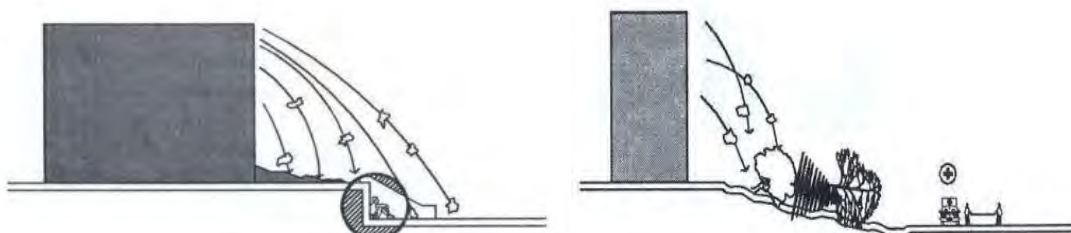
شکل ۵_ استفاده از اختلاف سطح جهت محافظت در برابر انفجار
