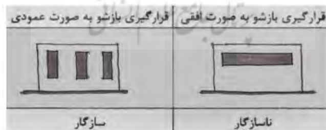
شکل ۱۶_ شیوه ی درست قرارگیری باز شوها، ماخذ: (ارشدی، ۱۳۹۱)
