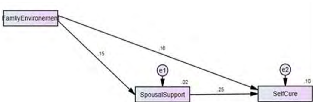
شکل ۲. مدل نهایی عوامل مؤثر بر مراقبت از خود بعد از انجام شاخص‌های برازش
