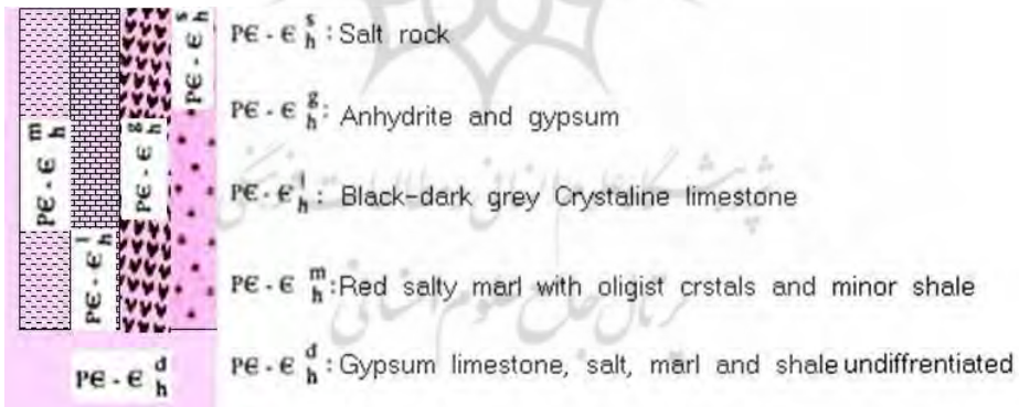
شکل ۳- ب- بارزسازی واحدهای سنگی سولفات (الف)، کربناته (ب)، رس (ج) و نمک (د) با پیکسل های روشن از دسته داده های AST_05 و نقشه زمین شناسی گنبد نمکی کنار سیاه (ه)
