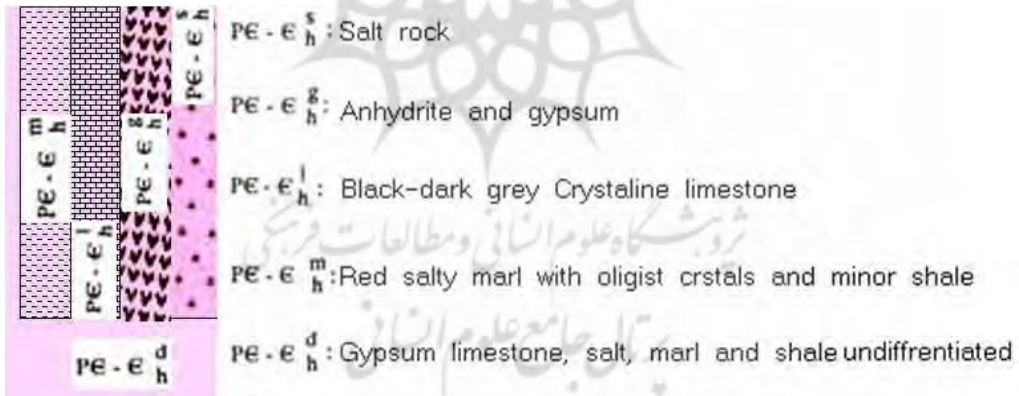
شکل ۳- الف- بارزسازی واحدهای سنگی سولفات (الف)، کربناته (ب)، رس (ج) و نمک (د) با پیکسل های روشن از دسته داده های AST_05 و نقشه زمین شناسی گنبد نمکی جهانی (ه)
