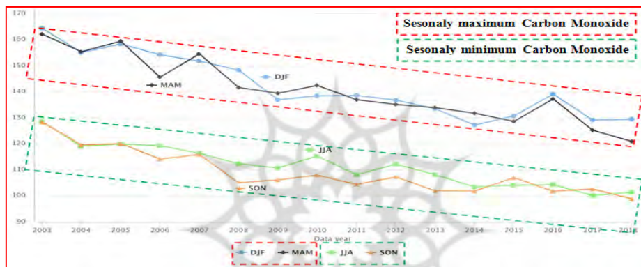
شکل ۸: سری زمانی تغییرات فصلی مونوکسید کربن سطحی بر فراز ایران (۲۰۱۸ - ۲۰۰۳)
