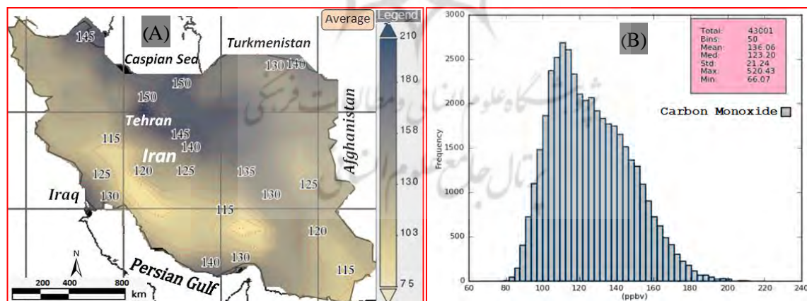
شکل ۱: (A) توزیع مکانی مونوکسید کربن سطحی و (B) توصیف آماری توزیع مونوکسید کربن سطحی و (A) توزیع مکانی مونوکسید کربن سطحی بر فراز ایران (۲۰۰۳ - ۲۰۱۸)
