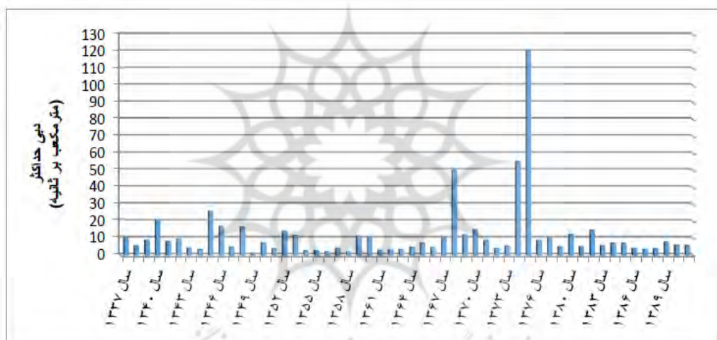
شکل ۶: نمودار دبی حداکثر سالانه ایستگاه تنگه لاویج رودخانه لاویج (دوره آماری ۱۳۳۷-۱۳۹۱)
