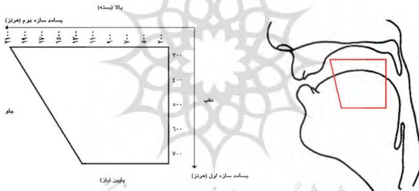
شکل ۱: نمایش فرضی فضای واکه‌ای در حفره دهان
