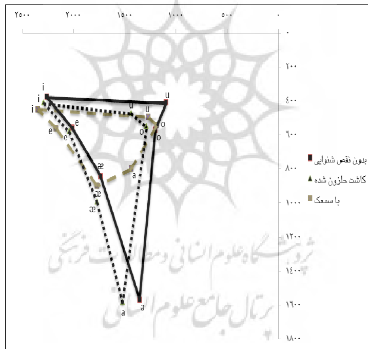
نمودار ۱۱: فضاهای واکه‌ای در کودکان دارای سمعک، کودکان کاشت حلزون شنوایی و کودکان بدون اختلال شنوایی
