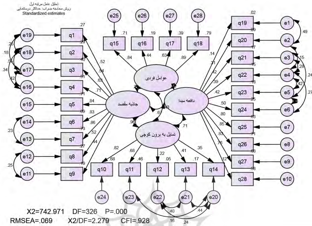
شکل ۱. مدل استاندارد معادله ساختاری تحلیل عاملی متغیرهای پژوهش
