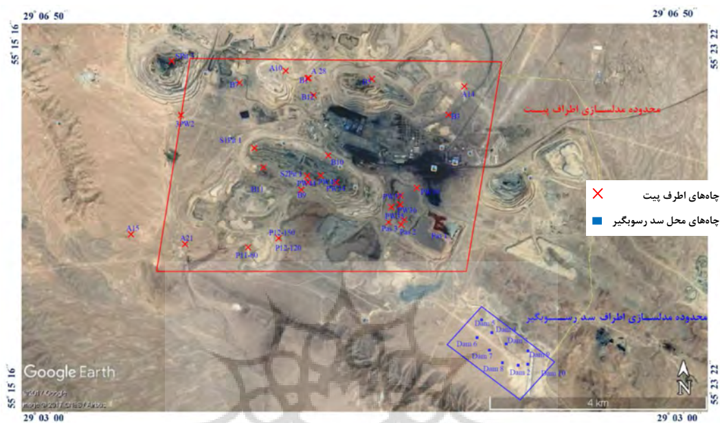
شکل ۳: محدوده‌ی مدل‌سازی اطراف بیت و سد رسوب‌گیر و موقعیت چاه‌های مشاهده‌ای
