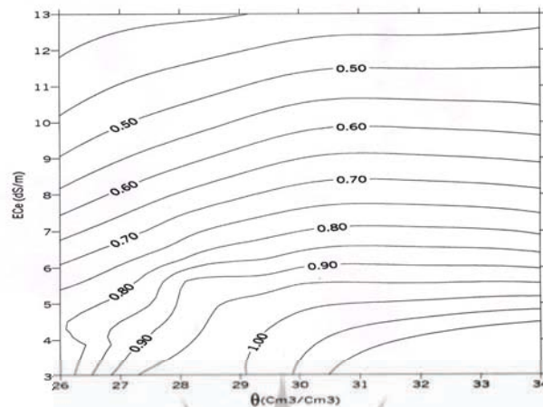
شکل ۲. منحنی هم‌محصول گندم تحت شرایط سطوح مختلف رطوبت و شوری خاک
