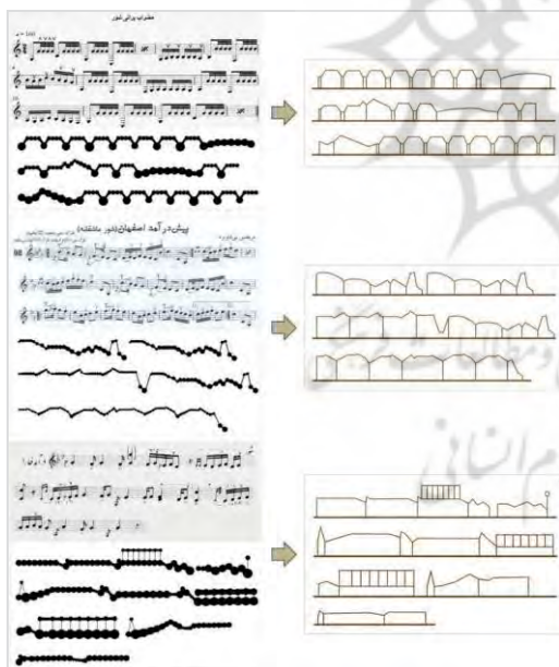
تصویر ۵- ترجمان تصویری بخشی از (۱) نت قطعه مضراب پرانی شور؛ (۲) وسط؛ پیش‌درآمد اصفهان؛ (۳) پایین: درآمد خارا؛ به صورت خطوط متشکل از نقاط به هم پیوسته (نگارندگان).
