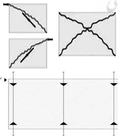
شکل ۴) بالا: دیوار بنایی غیرمسلح و ترک قطری در اثر کشش برشی ناشی از نیروی جانبی زلزله؛ پایین: مهاربندی دیوار خشتی مسلح توسط کابل های عمودی برای جلوگیری از ایجاد ترک قطری (ترسیم: نگارندگان)
