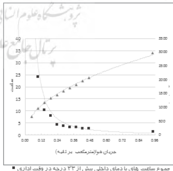
شکل ۷: مقایسه عملکرد برودتی و مصرف آب در دبی های مختلف جریان هوا (مأخذ: نگارندگان)
