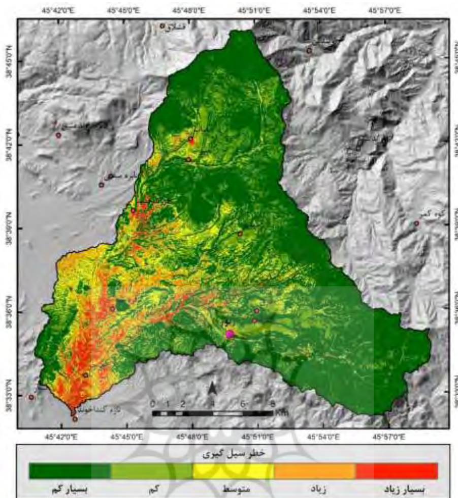
شکل ۸: پهنه‌بندی خطر سیل‌گیری حوضه آبریز زوزچای با استفاده از گامای فازی
