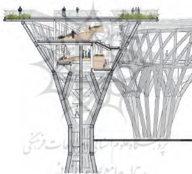
شکل ۷. برش عرضی پل طبیعت. مأخذ: Ettefagh & Ahmadi, 2017
