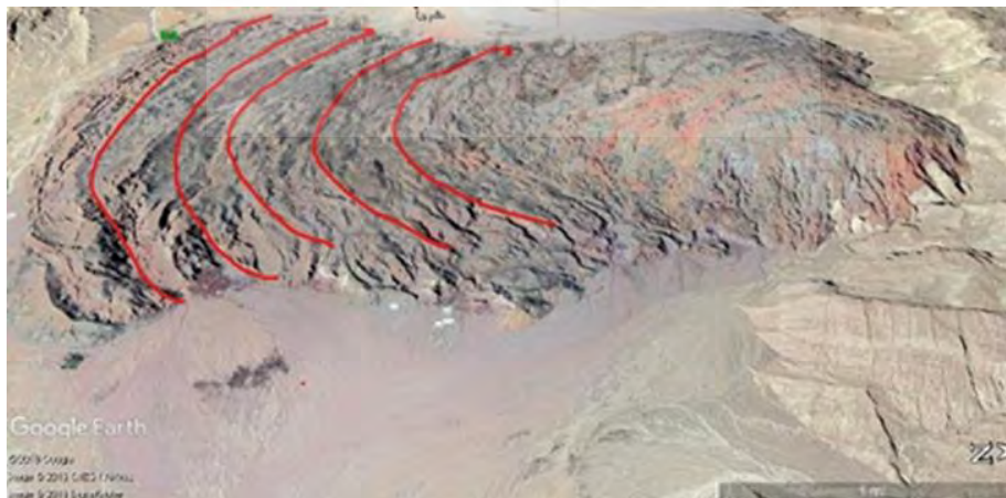
شکل ۵. خطوط عرضی سطح گنبد نمکی کرم‌سبز که حرکت نمک‌ها را نشان می‌دهد. جهت حرکت نمک عمود بر خطوط قرمز رنگ است.
