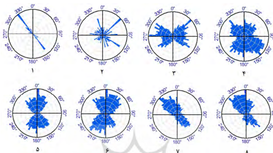
شکل ۲: نمودار رز خطواره‌ها: گسل‌ها ۱- به روش دستی، ۲- شبکه زهکشی، ۳- لندست ۸، ۴- تراسار x^1 (HH)، ۵- سنتینل ۱ ۲ بالاگذر، ۶- سنتینل ۱ پایین گذر، ۷- الوس پالساار (HV)، ۸- الوس پالساار (HH)
