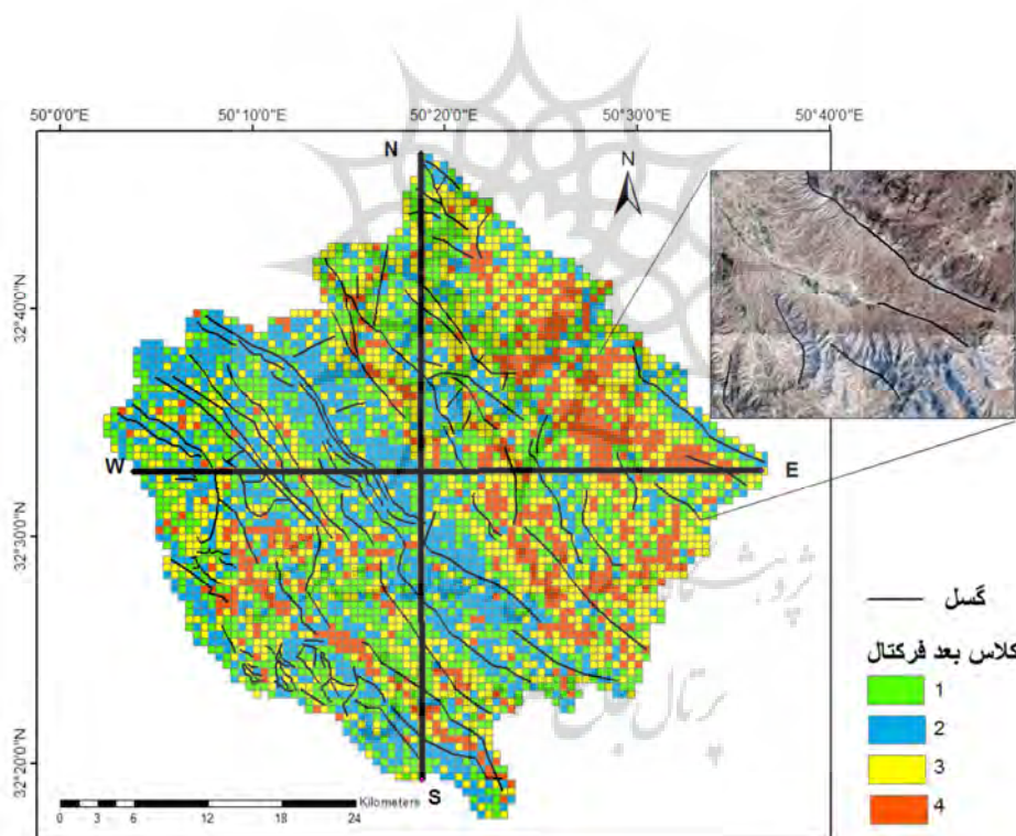
شکل ۴: نقشه توزیع بعد فرکتال حوضه و دو پروفیل شمال - جنوب و غرب - شرق
