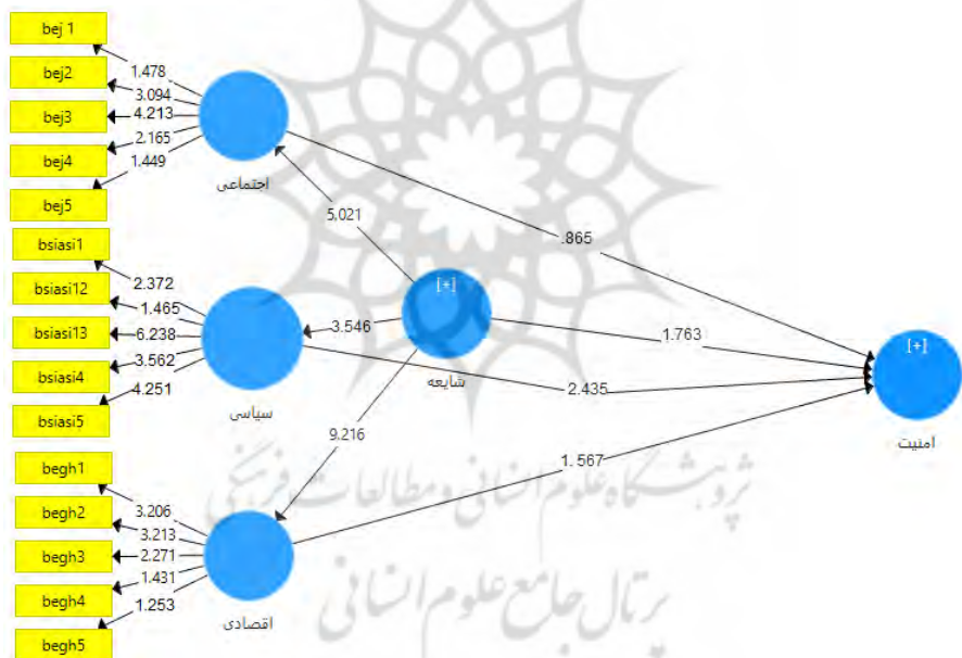
شکل ۲: آماره t-value
